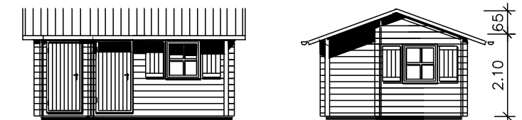
Ansichten First um 90° gedreht
