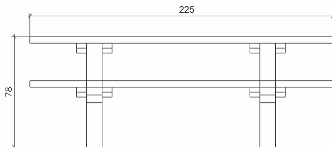
Systemzeichnung Typ SGD225
